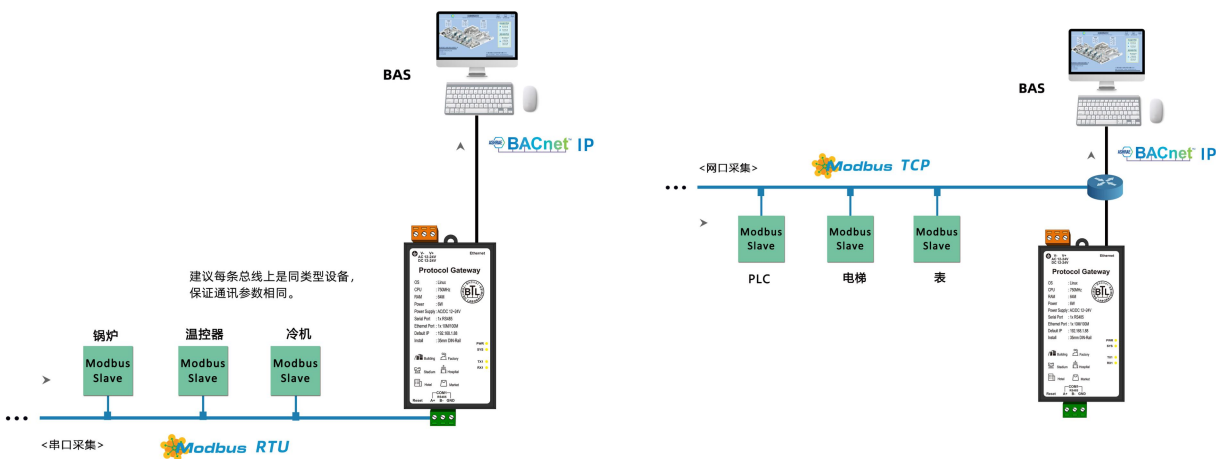
应用场景一：集成ModbusRTU转BACnet IP
