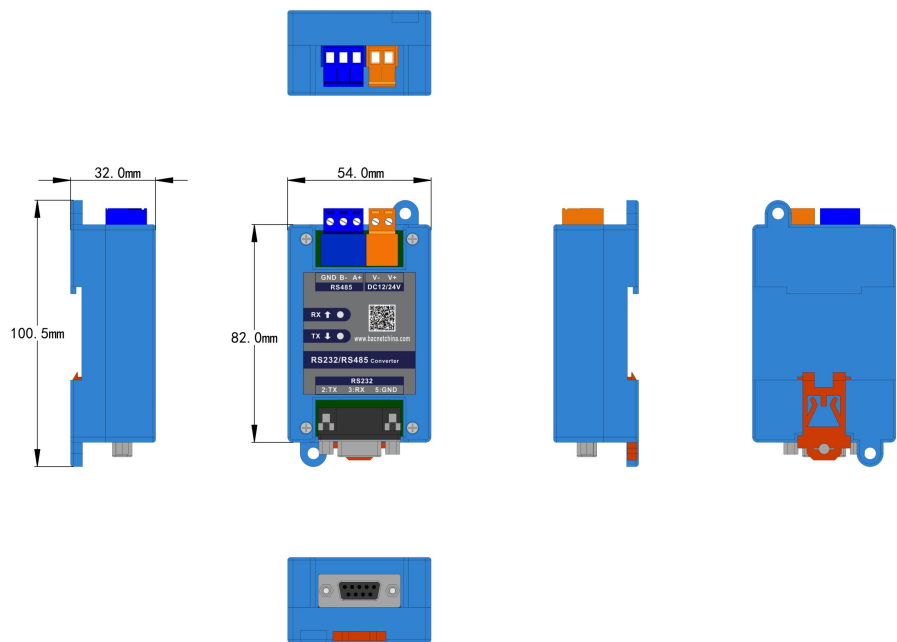
尺寸图
