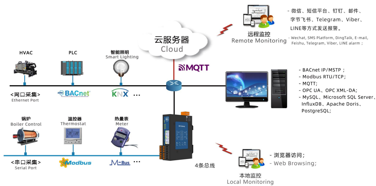
现场应用原理图
