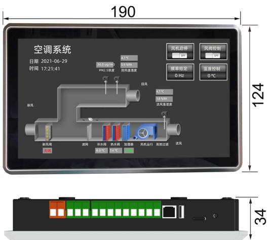
I7-1031产品尺寸
