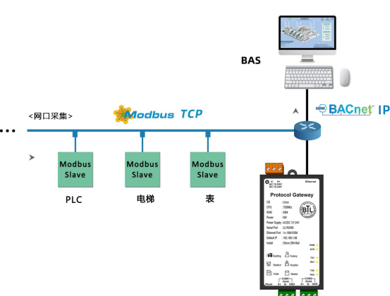
应用场景二：集成ModbusTCP转BACnet IP
