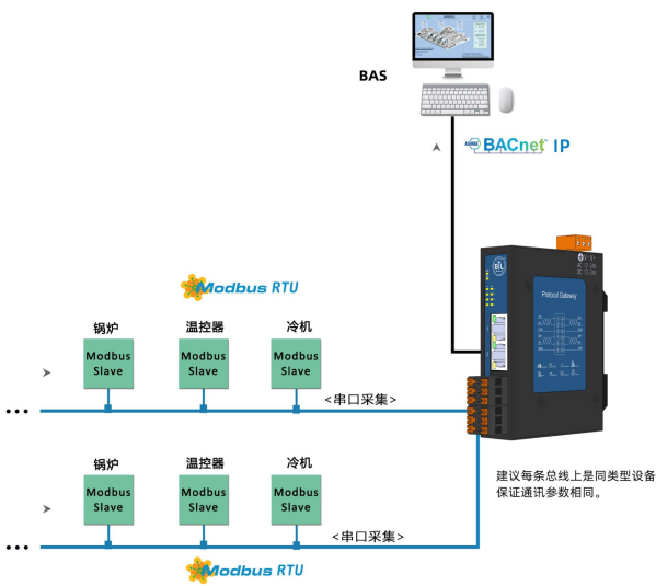
应用场景一：集成串口协议转BACnet IP
