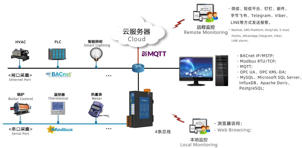
现场应用原理图
